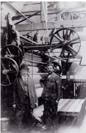
Afb. 2: weefgetouw aangedreven door een stoommachine in de fabriek in Goirle 2) . De man rechts op de foto is Harrie van Puijenbroek
